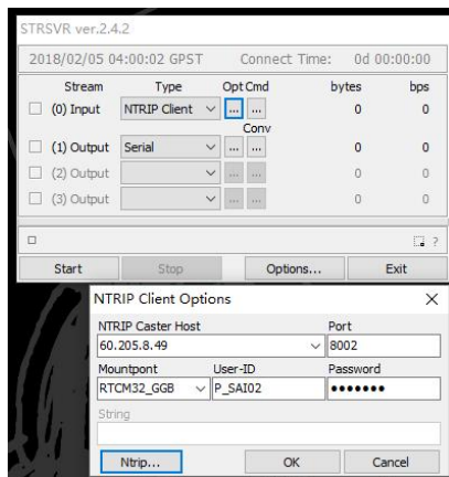
图 4.2 Ntrip Client 配置
