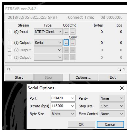
图 4.1 配置串口
