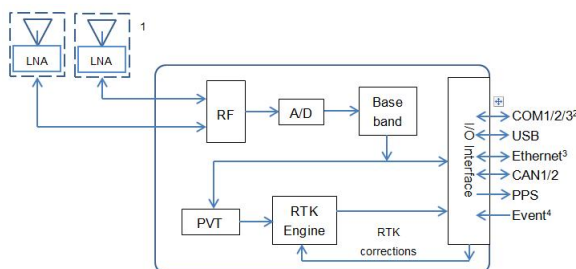
图 1.1 BX50L-TAP 系统概述
