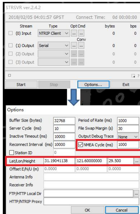
图 4.3 接收机位置配置
